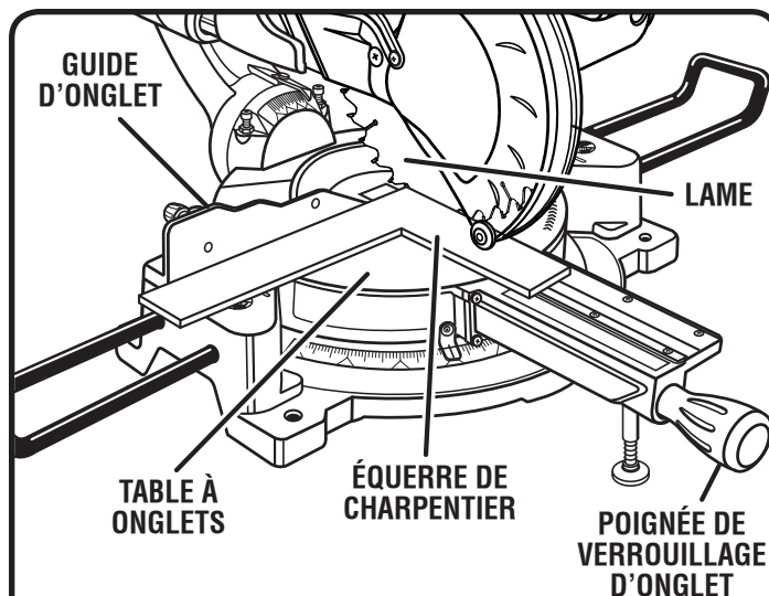
VUE DE LA LAME D'ÉQUERRE AVEC LE GUIDE
