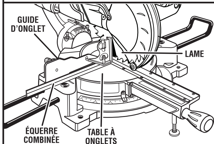
VUE DE LA LAME PAS D'ÉQUERRE AVEC TABLE À ONGLETS, DES RÉGLAGES SONT NÉCESSAIRES
