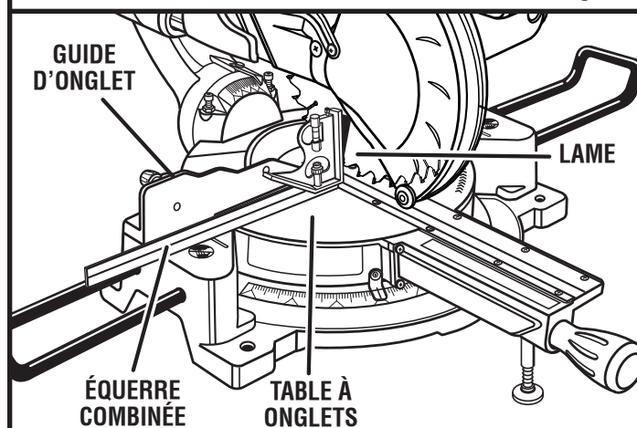
VUE DE LA LAME PAS D'ÉQUERRE AVEC LA TABLE, DES RÉGLAGES SONT NÉCESSAIRES
