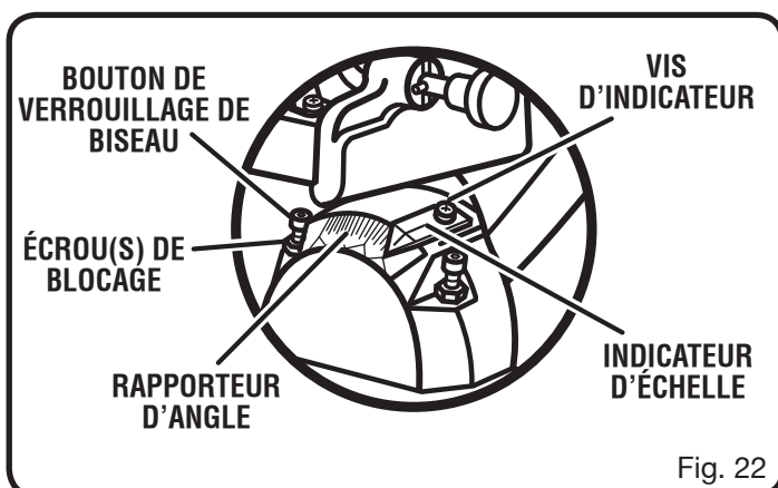
VUE DE LA LAME PAS D'ÉQUERRE AVEC TABLE À ONGLETS, DES RÉGLAGES SONT NÉCESSAIRES
