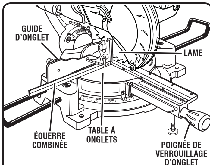
VUE DE LA LAME D'ÉQUERRE AVEC LA TABLE À ONGLETS
