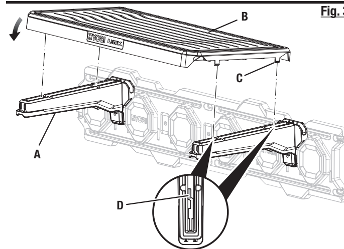
A - 2-in-1 shelving bracket (support d'étagère 2-en-1, soporte para estante 2 en 1) B - Solid shelf accessory (accessoire d'étagère solide, accesorio para estante sólido) C - Tab (languette, pestaña) D - Slot (fente, ranura)
