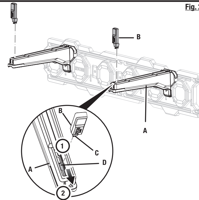
A - 2-in-1 shelving bracket (support d'étagère 2-en-1, soporte para estante 2 en 1) B - Material retention tab (languette de retenue du matériau, lengüeta de sujeción del material) C - Tab (languette, pestaña) D - Slot (fente, ranura)
