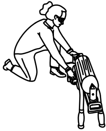
INCORRECT OPERATOR POSITION MAUVAISE POSITION D'UTILISATION POSICIÓN OPERATIVA INCORRECTA
