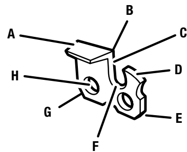
A - Top plate (plaque supérieure, placa superior) B - Cutting Corner (coupe de coin, esquina de corte) C - Side plate (plaque latérale, placa lateral) D - Depth gauge (limiteur de profondeur, calibre de profundidad) E - Toe (sabot, puntera) F - Gullet (creux, garganta) G - Heel (talon, talón) H - Rivet hole (trou de rivet, orificio del remache)
