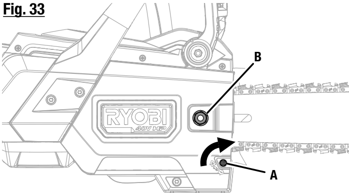
A - Chain tensioning screw (vis de tension de la chaîne, tornillo tensor de la cadena) B - Bar mounting nut (écrou de montage du guide, tuerca de montaje de la barra)
