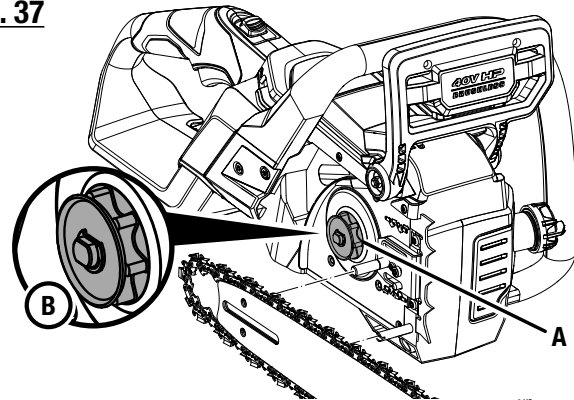
A - Drive sprocket (pignon d'entraînement, Rueda dentada de impulsión) B - Check for wear or damage (s'assurer de l'absence d'usure ou de dommages, revise para ver si hay desgaste o daños)
