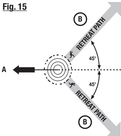
A - Planned line of fall (ligne de chute prévue, Línea de caída planificada) B - Straight arm position (chemin d'échappement, trayectoria de retirada)
