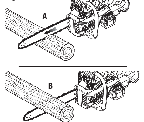
A - Overbucking (coupe par le dessus, tronzado por arriba) B - Underbucking (coupe par le dessous, tronzado por abajo)
