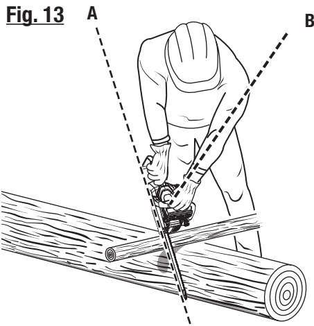
A - Chain line (ligne de chaîne, plano de la cadena) B - Straight arm position (bras tendu, posición con el brazo recto)
