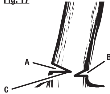
A - Back cut (entaille d'abattage, corte trasero) B - Notch (encoche, muesca) C - Hinge charnière, bisagra
