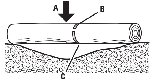
A - Load (charge, carga) B - 1st cut - 1/3 diameter (1ère coupe 1/3 diam, primer corte, 1/3 del diám.) C - Finishing cut (coupe de finition, corte final)
