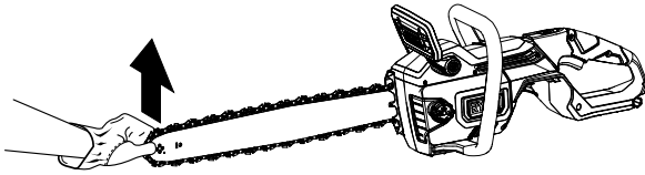
Fig. 32 LIFT THE TIP OF THE GUIDE BAR UP TO CHECK FOR SAG RELEVER L'EXTRÉMITÉ DU GUIDE POUR VÉRIFIER LE MOU LEVANTE LA PUNTA DE LA BARRA GUÍA PARA REVISAR LA HOLSURA DE LA CADENA
