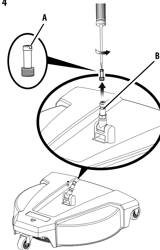
A - High pressure filter (filtre haute pression, filtro de alta presión) B - Cleaning deck inlet plug (prise de nettoyer le filtre d'arrivée d'eau, clavija de entrada de la unidad de limpieza)
