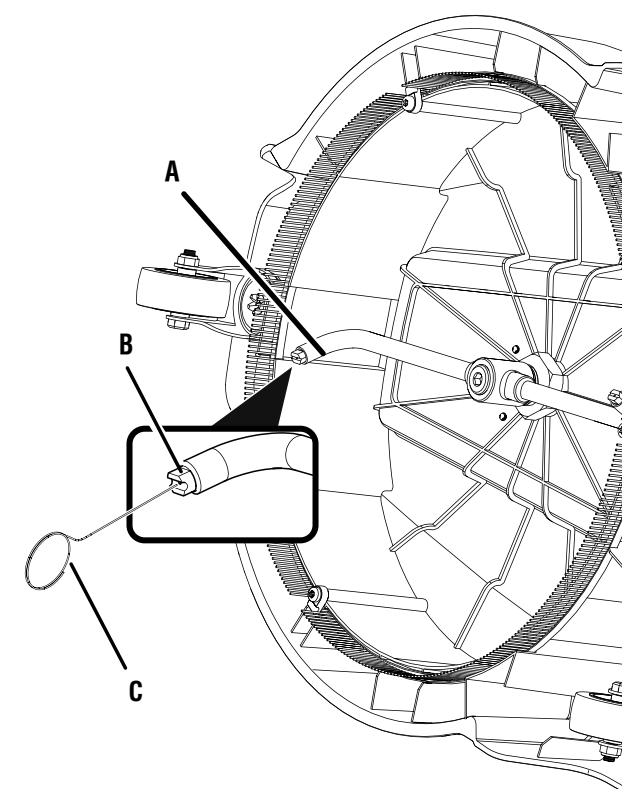
A - Spray bar (barre de pulvérisation, tubo rociador) B - Nozzle (buse, boquilla) C - Nozzle cleaning tool (nettoyer les buses, herramienta para limpiar boquillas)
