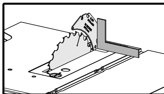
AJUSTE VERTICAL
