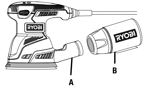
A - Dust exhaust (sortie de poussière, escape de polvo) B - Dust bag assembly (sac à poussière, conjunto del saco captapolvo)
