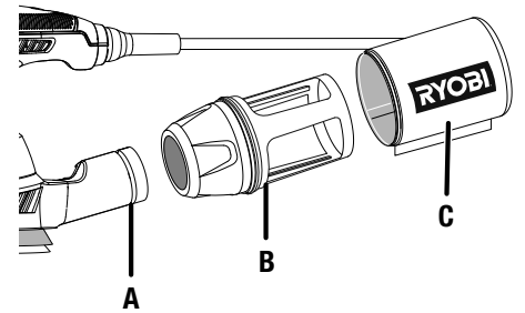
A - Dust exhaust (sortie de poussière, escape de polvo) B - Frame (support, armazón) C - Dust bag (sac à poussière, saco captapolvo)
