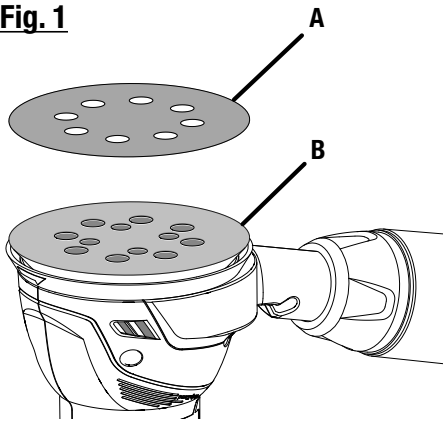
A - Hook-and-loop sanding disc (disque abrasif à boucles et crochets, disco de lija de gancho y lazada) B - Backing pad (coussinet, almohadilla de respaldo)
