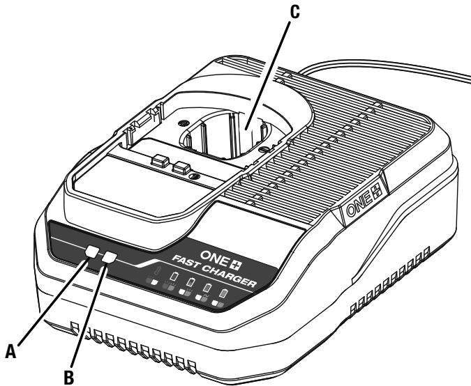
A - Red LED (témoin rouge, indicador de rojo) B - Green LED (témoin vert, indicador de verde) C - Battery port (port de pile, port de batería)
