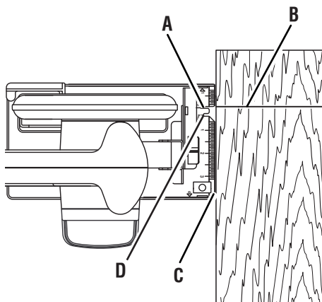
Fig. 14 TOP VIEW OF SAW (VUE SUPÉRIEURE DE SCIE, VISTA SUPERIOR DE LA SIERRA)
