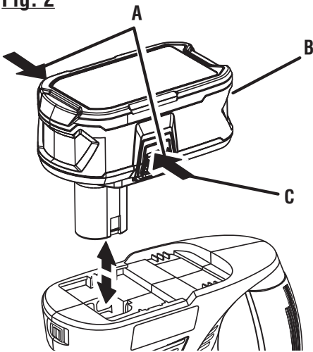
A - Depress latches to release battery pack (appuyer sur les loquets pour libérer le bloc-pile, para soltar el paquete de baterías oprima los pestillos) B - Battery pack (bloc-pile, paquete de baterías) C - Latches (loquets, pestillos)
