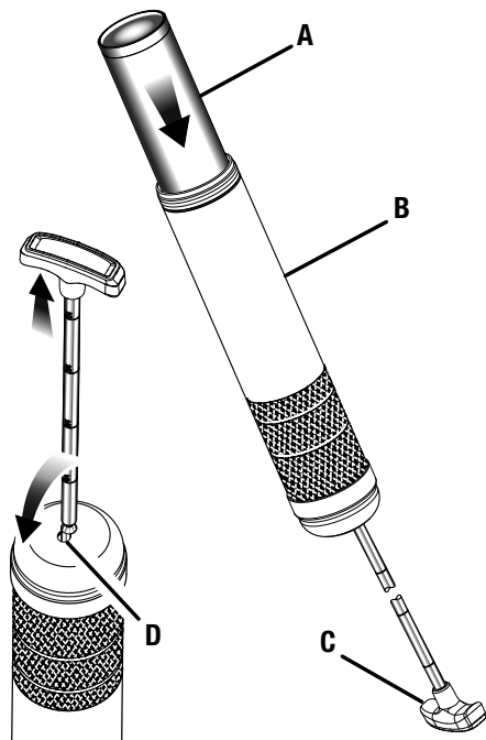
A - Grease cartridge (not provided) [cartouche de graisse (non comprise), cartucho de grasa (no incluido)] B - Grease tube (tube de graisse, tubo de grasa) C - Grease tube handle (poignée du tube de graisse, mango del tubo de grasa) D - Narrow slot (fente étroite, ranura estrecha)
