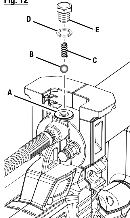
A - Check valve area (zone du clapet antiretour, área de la válvula de retención)
