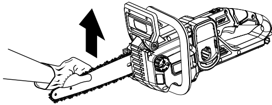
Fig. 29 LIFT THE TIP OF THE GUIDE BAR UP TO CHECK FOR SAG RELEVER L'EXTRÉMITÉ DU GUIDE POUR VÉRIFIER LE MOU LEVANTE LA PUNTA DE LA BARRA GUÍA PARA REVISAR LA HOLSURA DE LA CADENA
