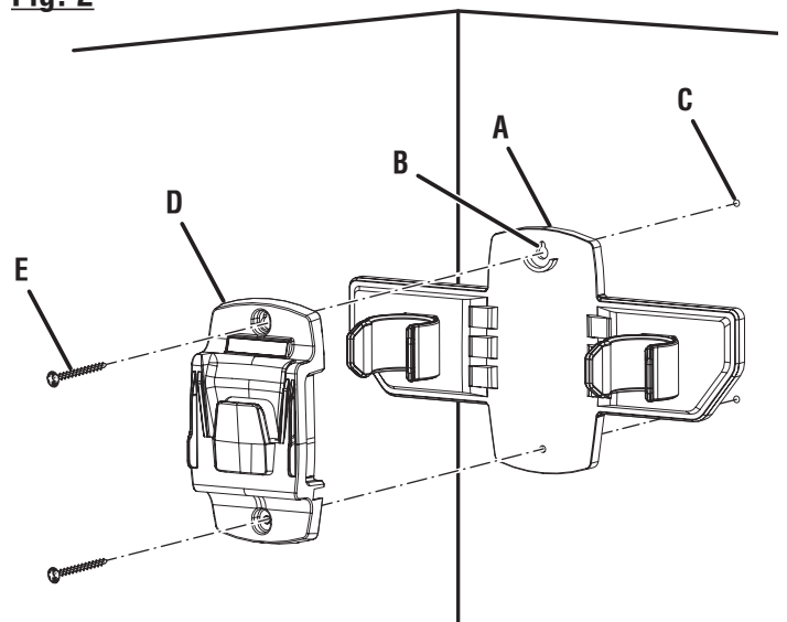
A - Optional accessory holder (support pour accessoires en option, soporte opcional para accesorios) B - Key hole hanger (trou de serrure pour la suspension, colgador tipo bocallave) C - Screw hole (orifice de las vis, agujero del tornillo) D - Cradle (logement, receptáculo) E - Screw (vis, tornillo)
