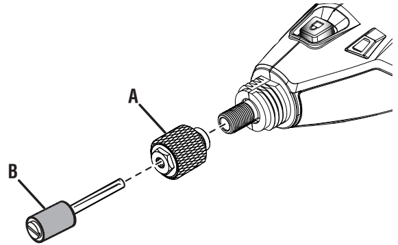
A - Quick-change collet (collet à changement rapide, portabroca de cambio rápido)
