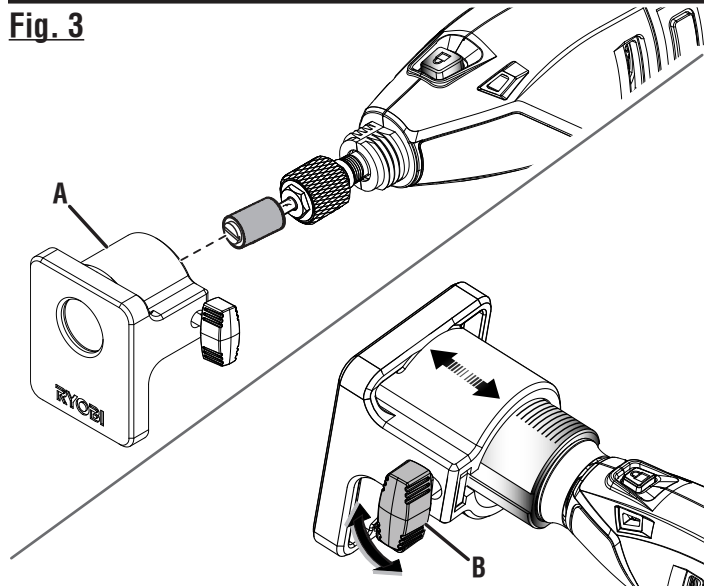
A - Attachment head (tête de l'accessoire, cabezal del accesorio)
